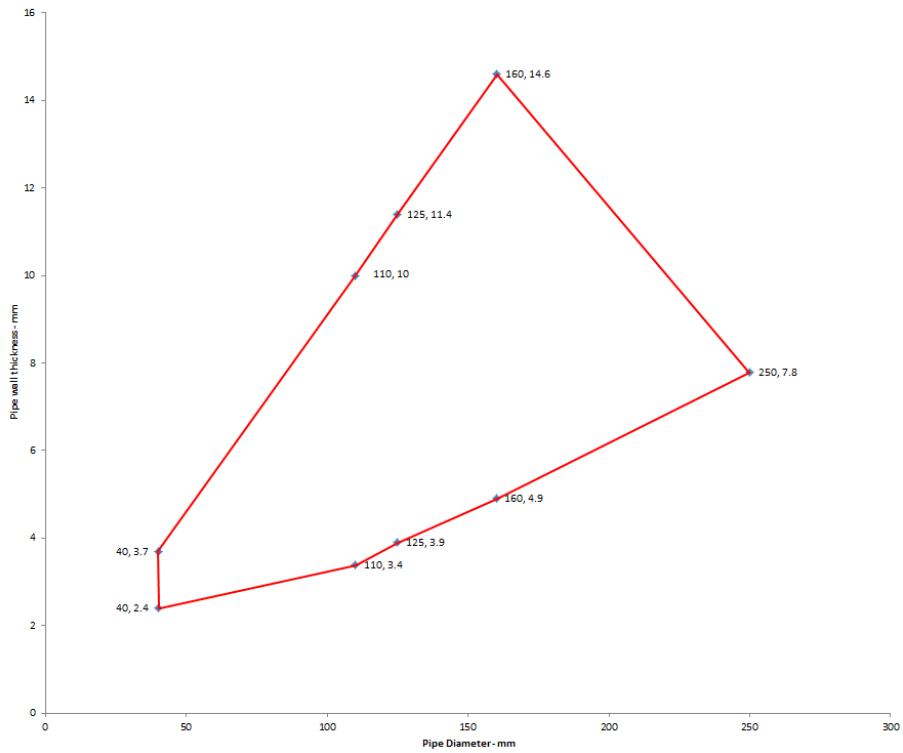
PE pipes U/C with FP Pipe Wrap/Rørstruper - EI 120 U/C
